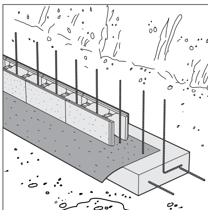
Kuva 8. Ensimmäinen harkkokerros.
