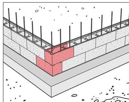
Kuva 9. Ladottaessa kulmaharkkojen välille syntyvä nurkkalukitus.
