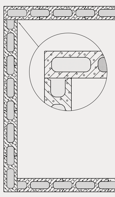
Parilliset harkkokerrokset
