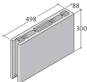
Leca® EasyLex 88 VS pääty *)
